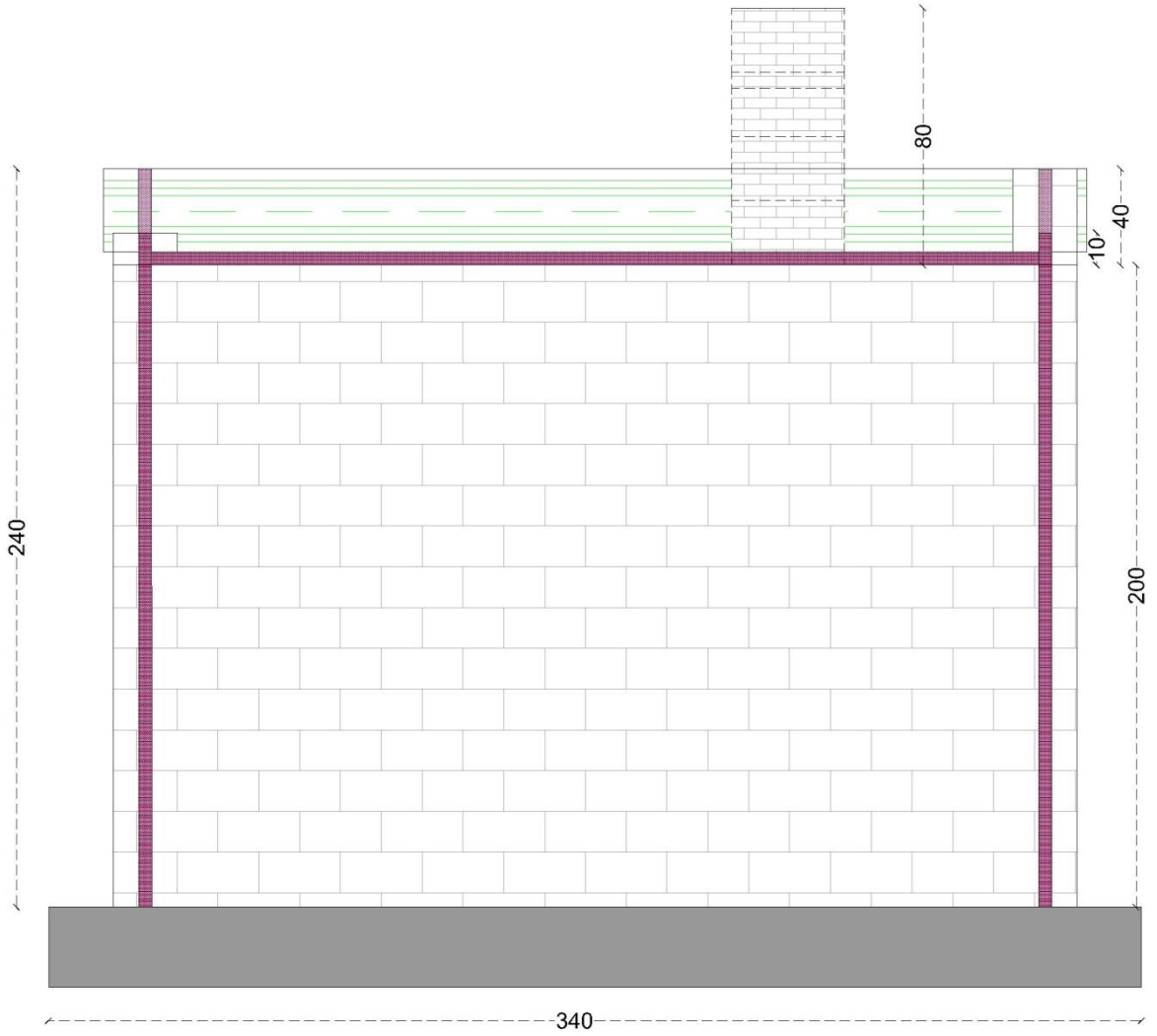
Arka Görünüş
